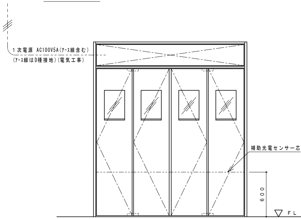
*内観図 (両折り戸)
