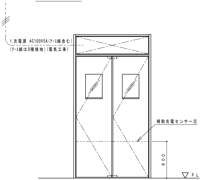
*内観図 (片折り戸)
